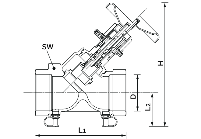
V5032...B Kombi-2-plus (DN65 - DN80)
