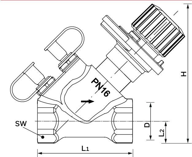
V5032...B Kombi-2-plus (DN15 - DN50)
